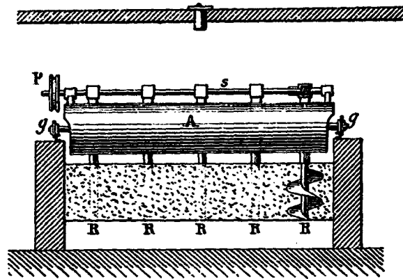
Fig. 69. — Coupes longitudinale et transversale d'une case de germination pneumatic (système Saladin).
