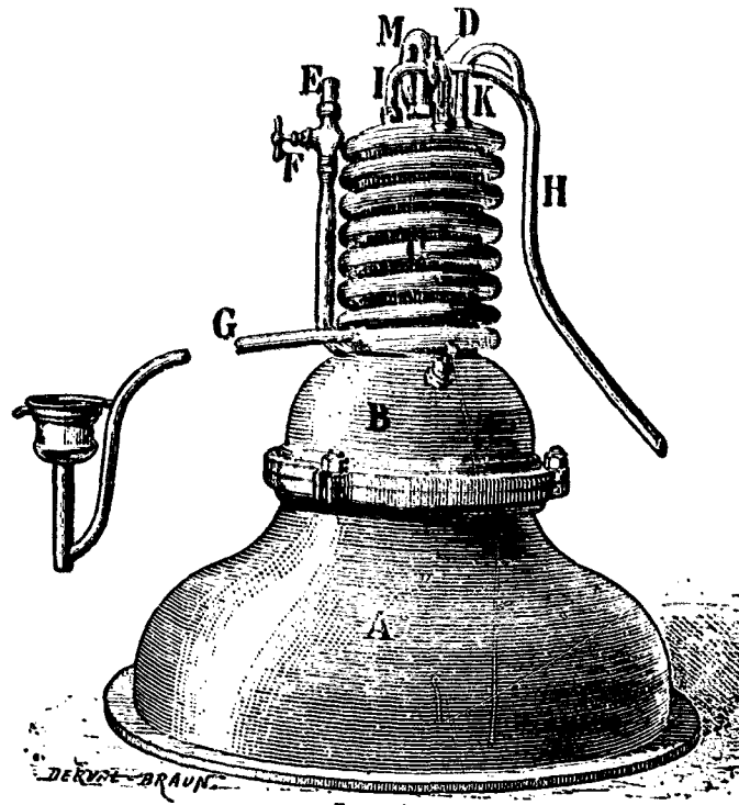
Fig. 53. — Appareil Lavy.
