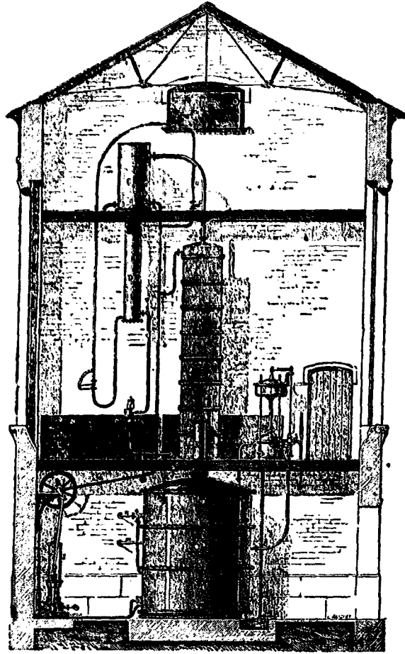
Fig. 31. — Rectificateur Savalle à colonne rectangulaire.
