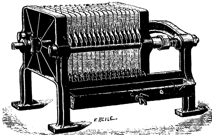
Fig. 81. — Filtre-presse.
