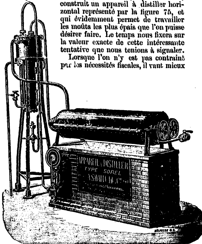
Fig. 75. — Appareil à distiller horizontal de M. Sorel.
