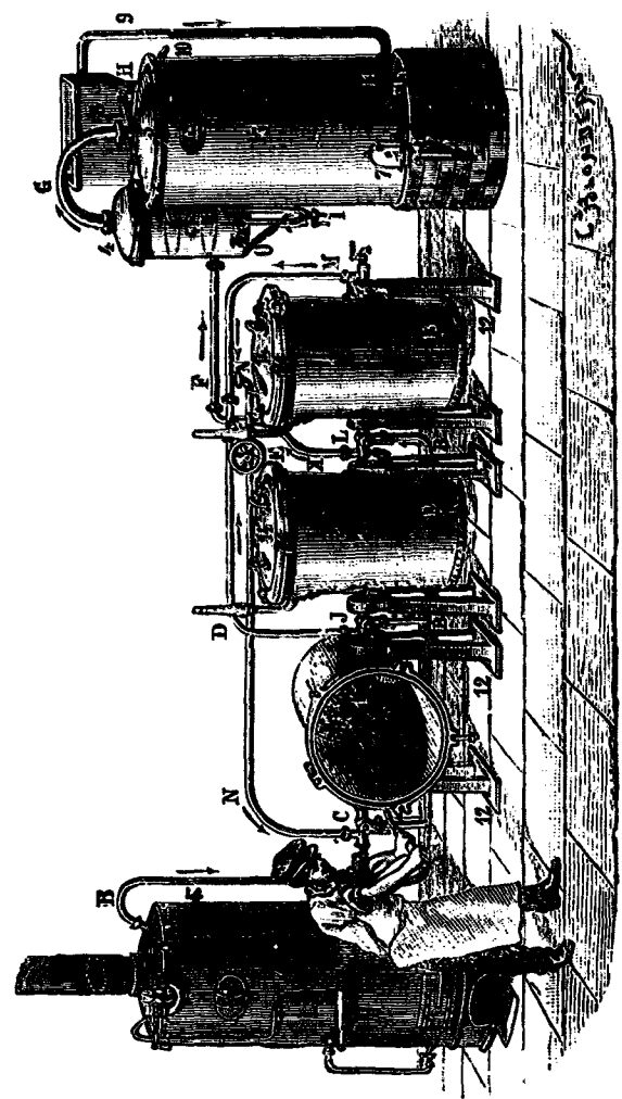
Fig. 51. — Appareil à distiller les marcs, système Peroy.
