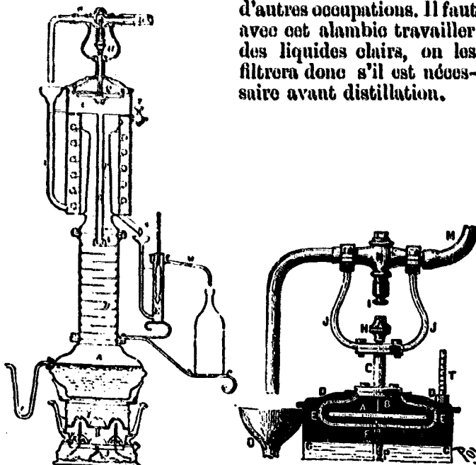
Fig. 45. — Alambic Besnard.
