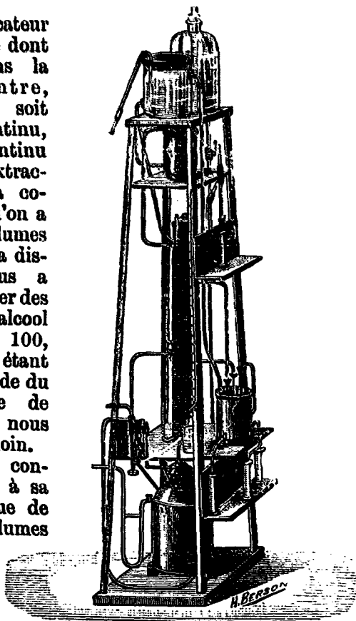
Fig. 4. — Rectificateur de laboratoire, système E. Barbet.
