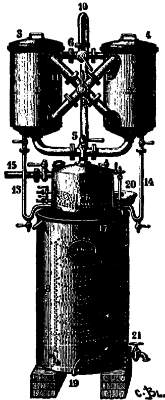
Fig. 84. — Anisateur continu, système Deroy.
