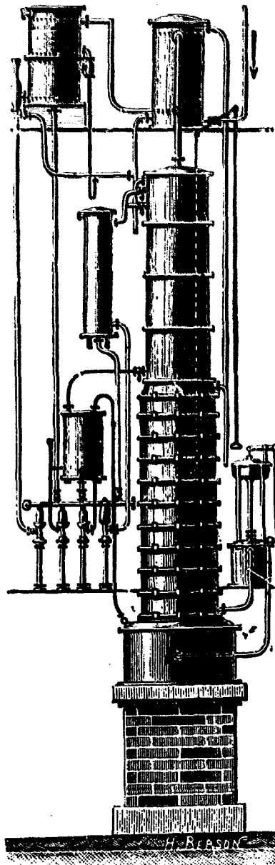
Fig. 38. — Colonne rectificatrice simple.
