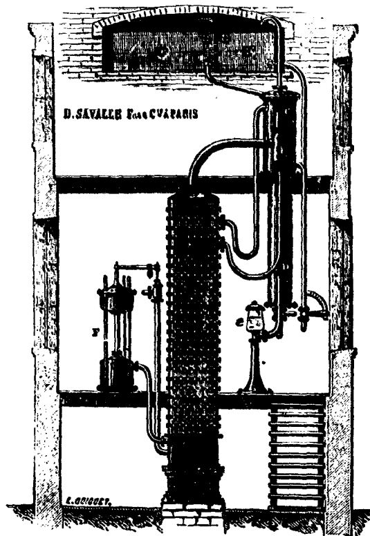
Fig. 25. — Colonne à distillation continue, système Savalle.
