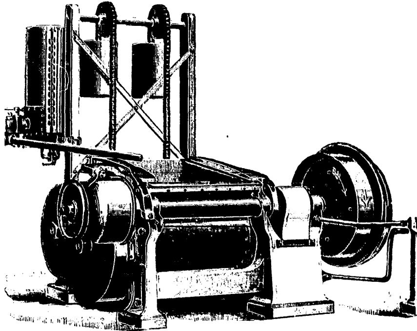
Fig. 83. — Pétrisseur pour l'empâtage des levains, système Werner et Pfleiderer.
