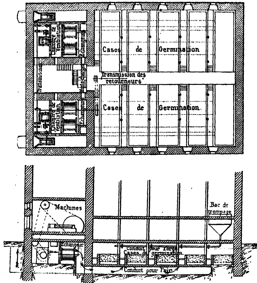
Fig. 70. — Plan et coupe verticale d'une installation pneumatique (système Saladin).
