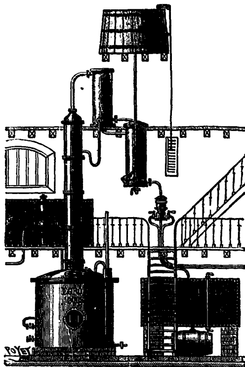
Fig. 30.— Colonne à rectifier discontinue, système Egot
