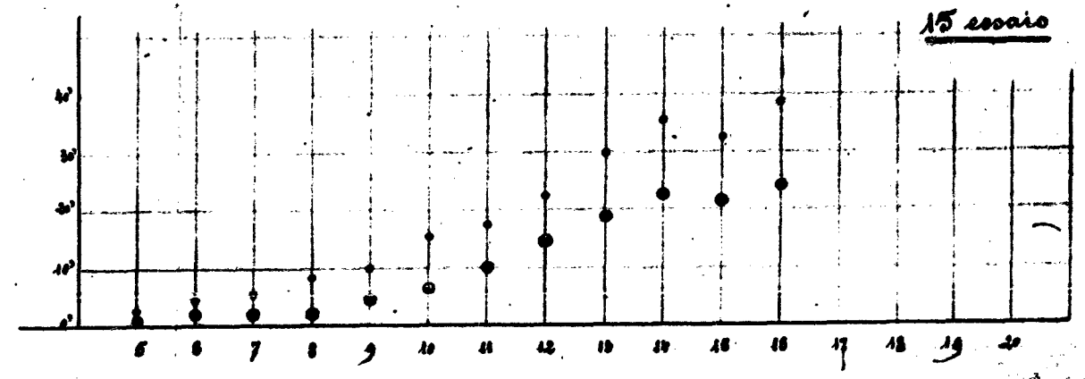
Fig VIII Série tirée d'une Rectification d'alcool brut de mélasse
