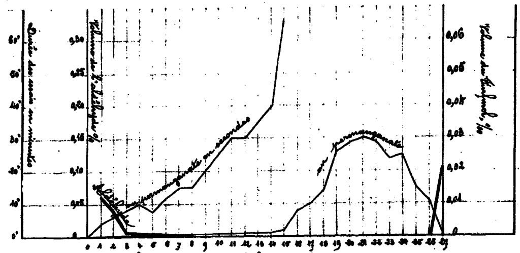
Rectification d'alcool brut de Pommes de terre et de Fruits à pépins
