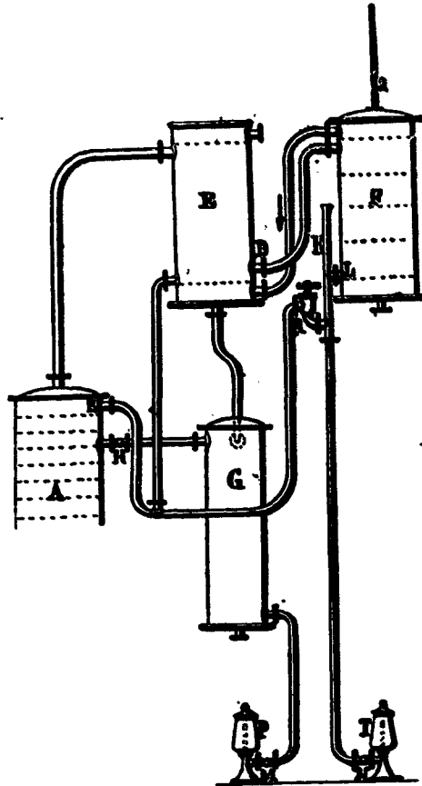
Fig. 35. — La Pasteurisation et le Réglage invariable du coulage. A, plateaux de rectification. — E, condenseur. — F, Réfrigérant. — L, Sortie de l'alcool froid. — K, trompette d'air. — T, éprouvette de l'alcool de tête. — N, robinet réglant le coulage invariable. — H, clapet de retenue laissant retourner à la rétrogradation B l'excès d'alcool de tête. — H, robinet d'extraction d'alcool pasteurisé. — G, réfrigérant du pasteurisé. — M, robinet réglant le coulage du pasteurisé. — P, éprouvette.
