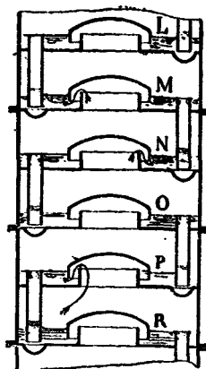
Fig. 24. Schéma de la colonne à plateaux.
