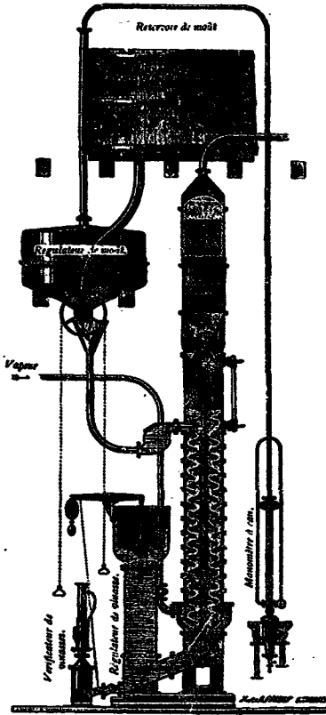
Fig. 37. — Colonne Ilgès.
