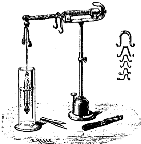
Fig. 1. — Balance hydrostatique de Mohr. accompagnent chaque appareil nous dispensent d'autres explications.
