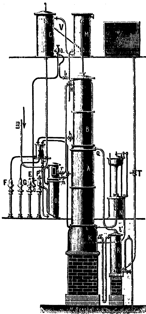
Fig. 48. — Colonne à pasteurisation pour eaux-de-vie et rhums.
