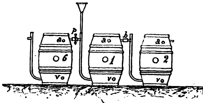
Fig. 50. — Diffusion des marcs.
