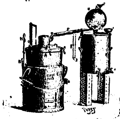
Fig. 52. — Alambic Egrot.
