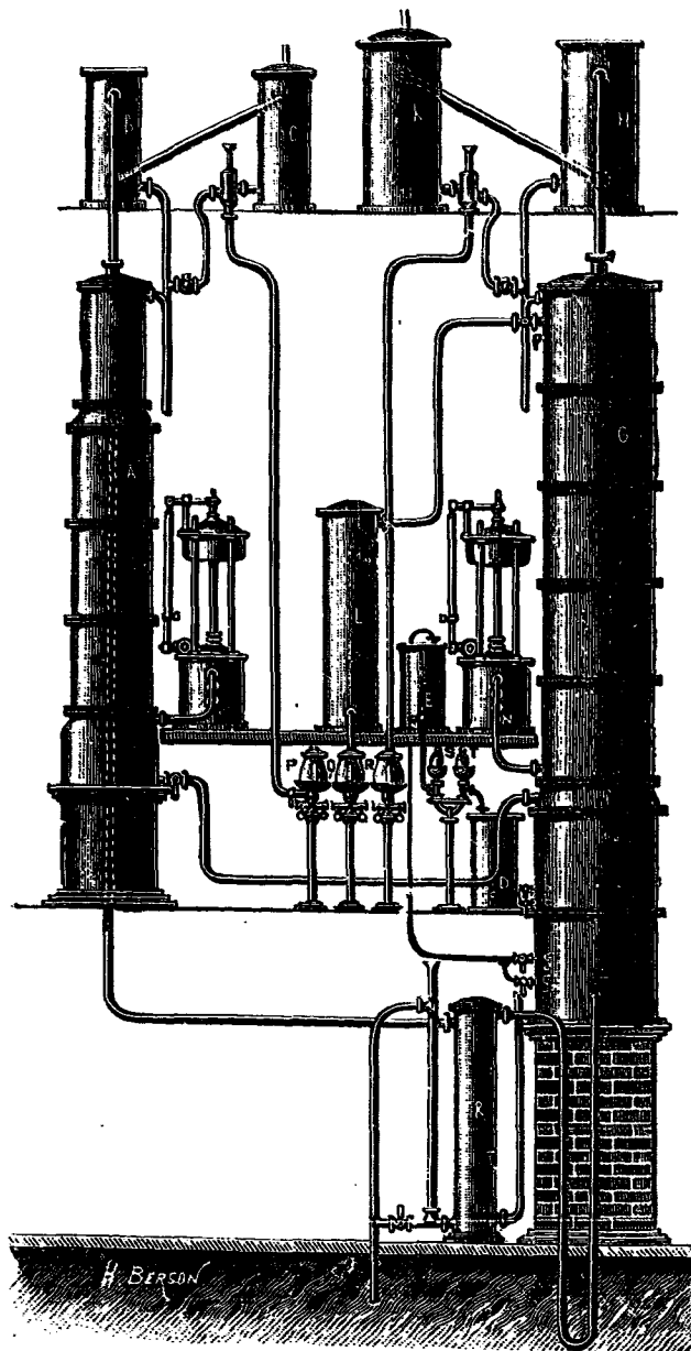
Fig. 34. — Rectificateur continu, système E. Barbet.
