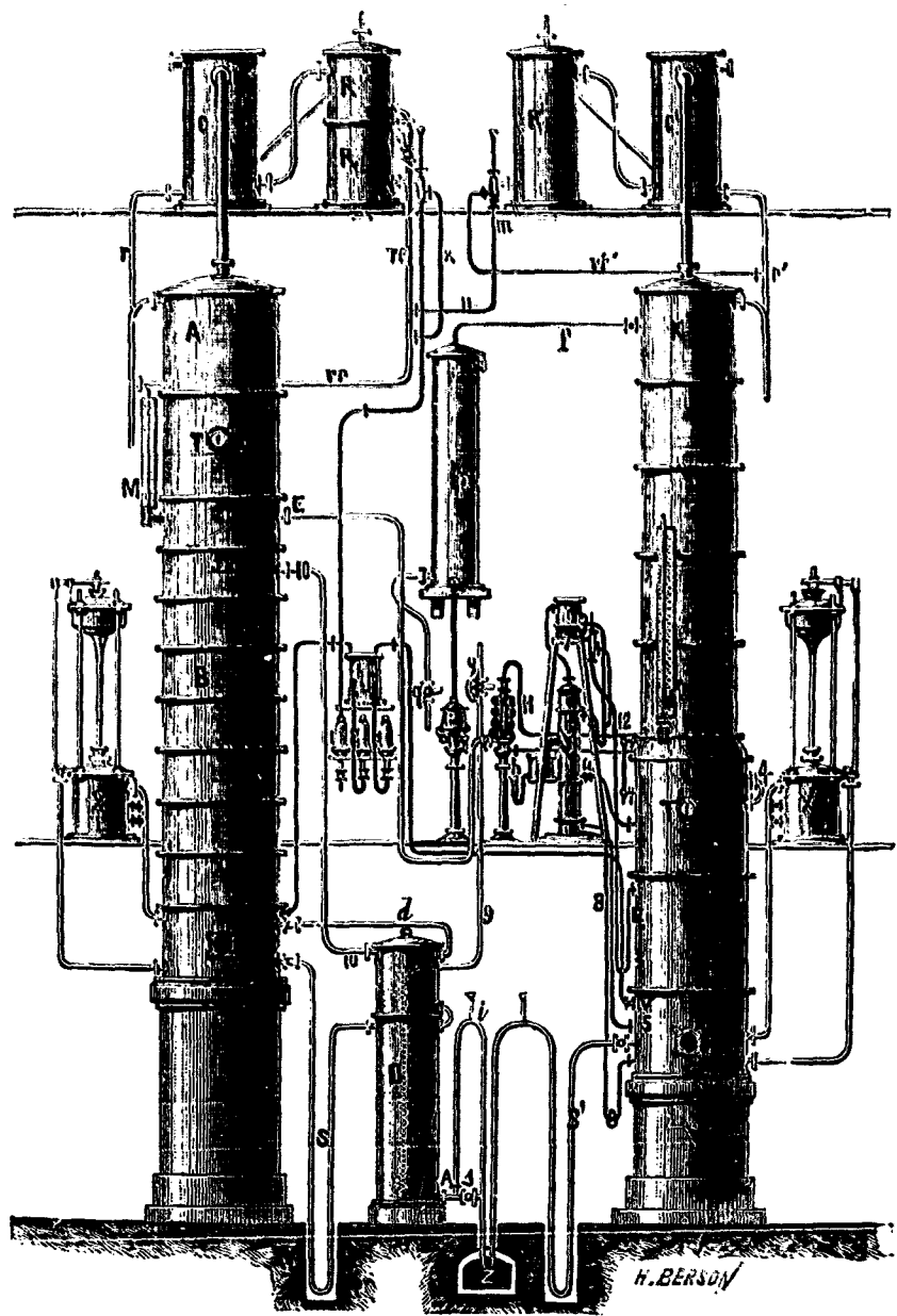
Fig. 40. — Colonne rectificatrice jumelle.
