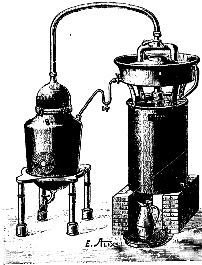
Fig. 44. — Alambic Bréhier chauffé par la vapeur.
