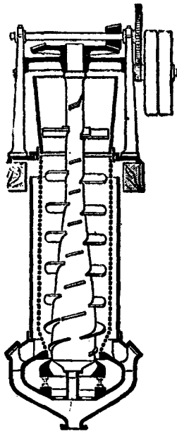
Fig. 58. Presse Klusemann.
