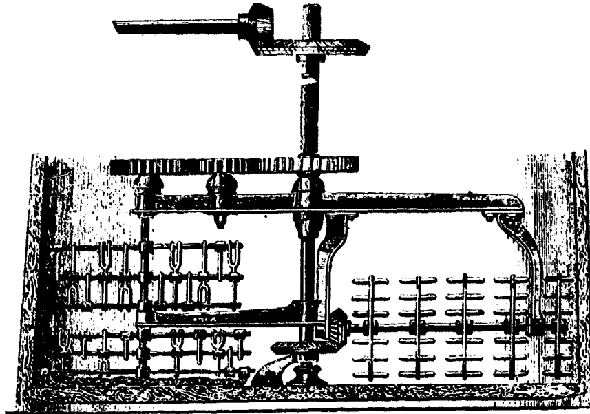
Fig. 77. — Macérateur ou cuve-matière.
