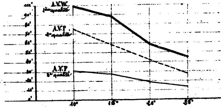
Fig. IX Influence de la température sur les essais au permanganate de potasse
