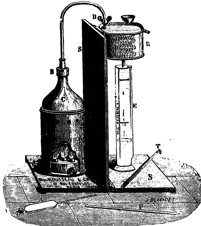
Fig. 3. — Alambic pour l'essai des vins.
